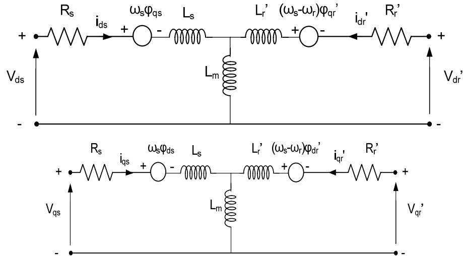
Figure 8: Schéma équivalent de la machine asynchrone selon l'axe "d" et l'axe "q"
